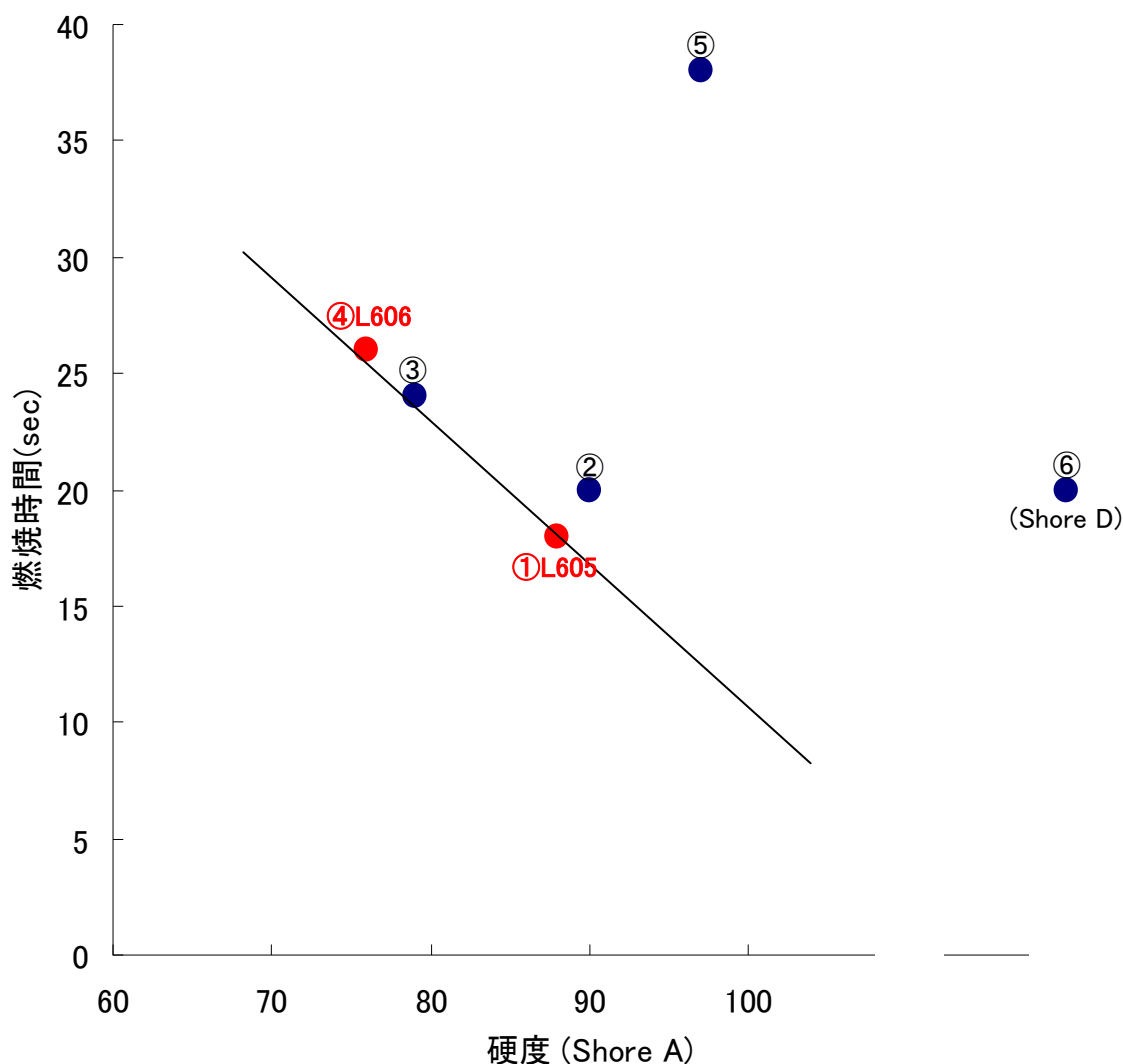
図3: PPE樹脂/S.O.E.® or SEBS/リン系難燃剤 組成物の硬度と燃焼時間の関係
